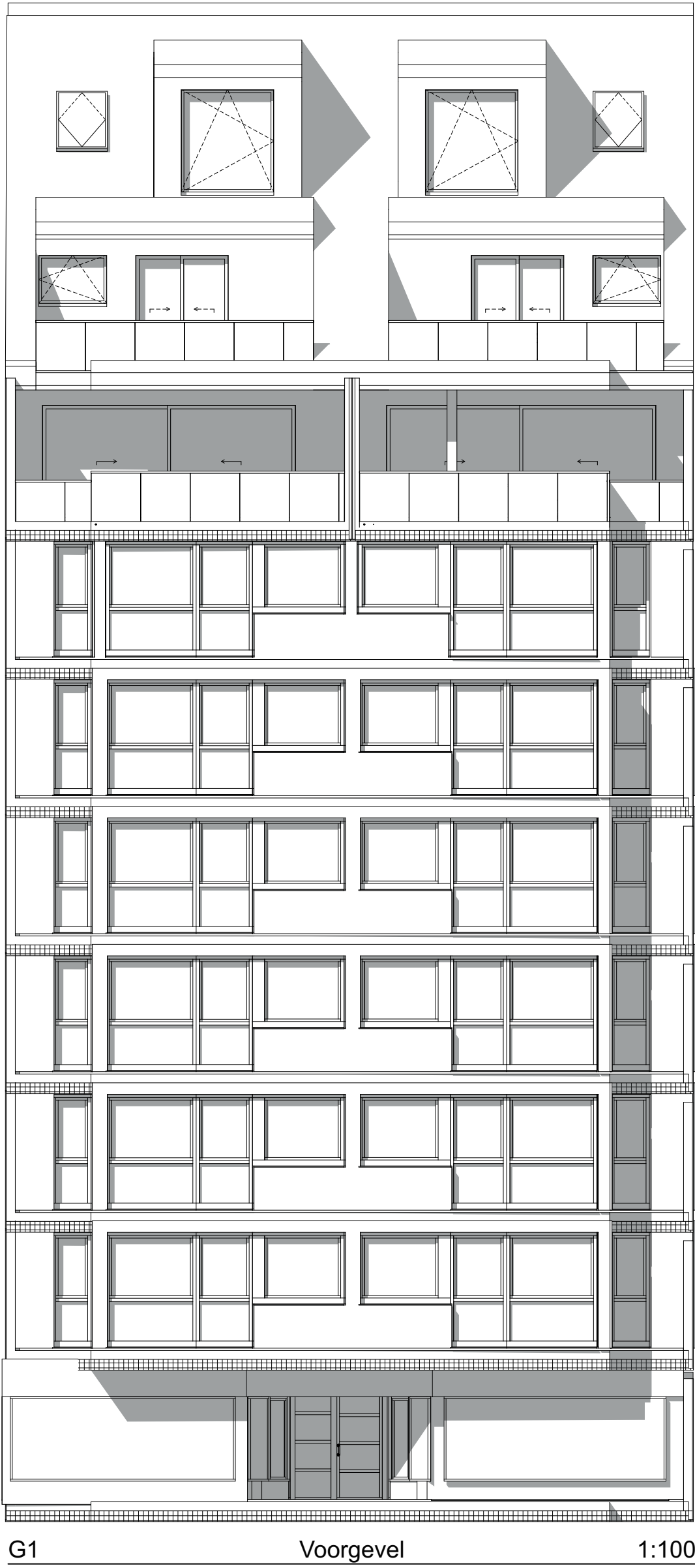
G1 Voorgevel 1:100
