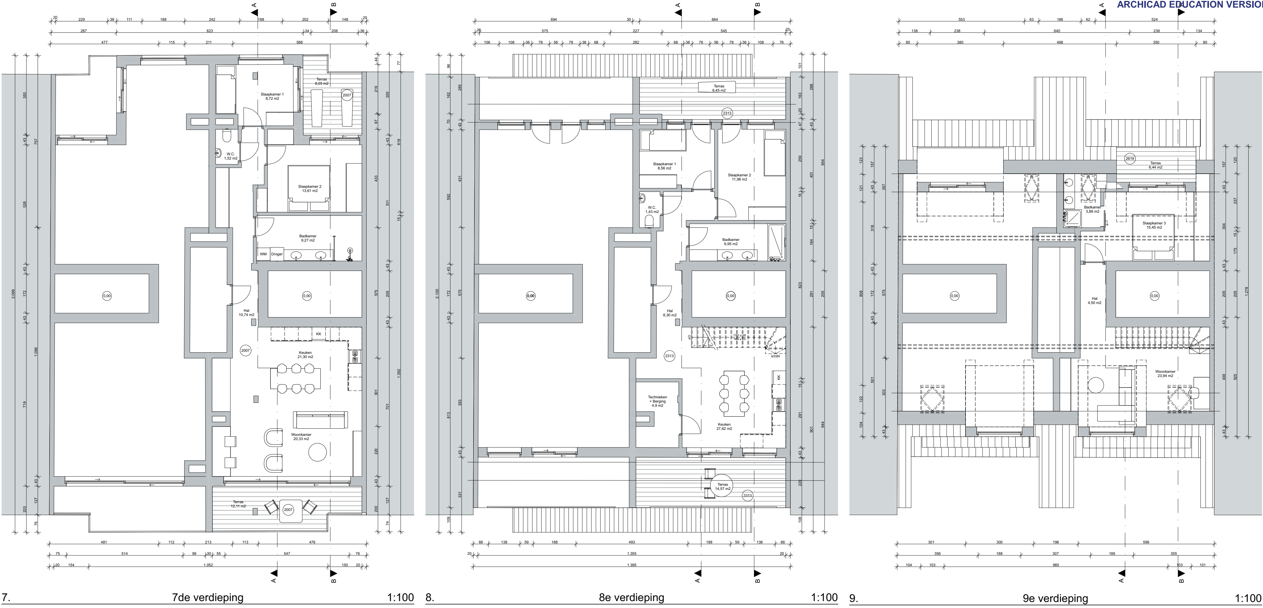
7. 7e verdieping 1:100 8. 8e verdieping 1:100 9. 9e verdieping 1:100
