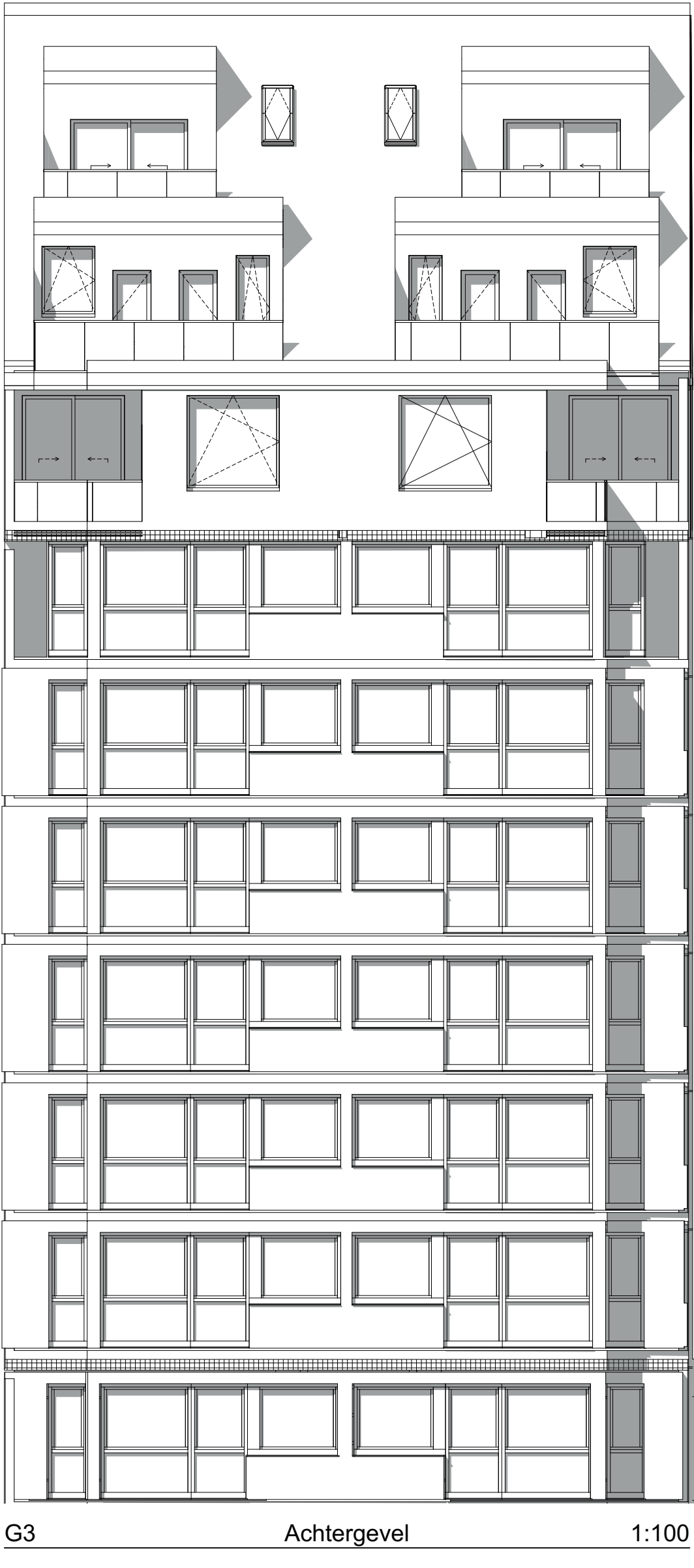
G3 Achtergevel 1:100
